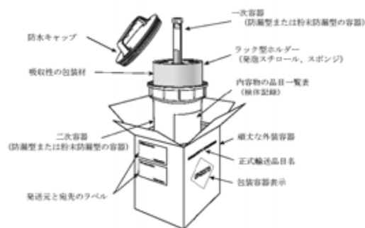
図 9: カテゴリーBの感染性物質の三重包装手法の包装容器とラベル貼付の例 (図は IATA [カナダ、セントリオール] の提供)
