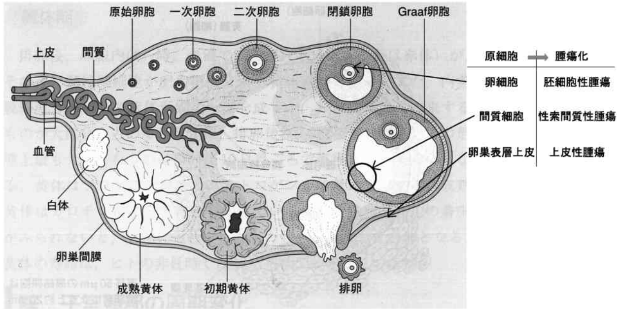
図1 卵巣の解剖
