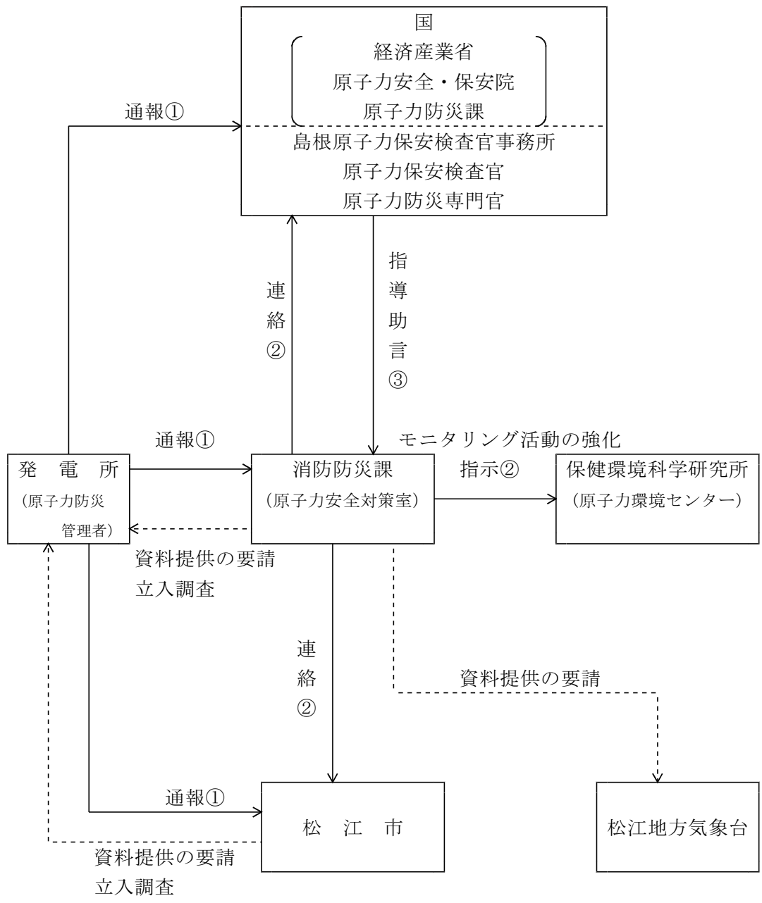
発電所異常時連絡系統図
